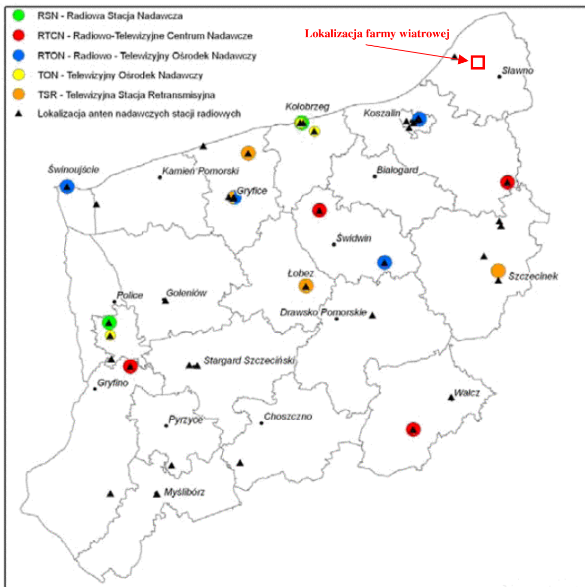
Rys. 6. Lokalizacja nadajników radiowo-telewizyjnych w kontekście lokalizacji farmy wiatrowej Boryszewo III
