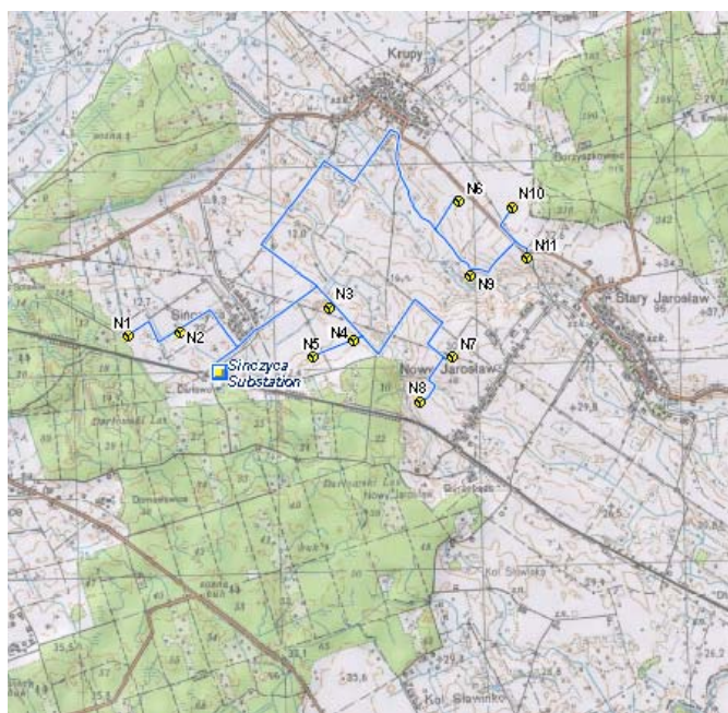
Rys.1. Farma wiatrowa Nowy Jarosław
